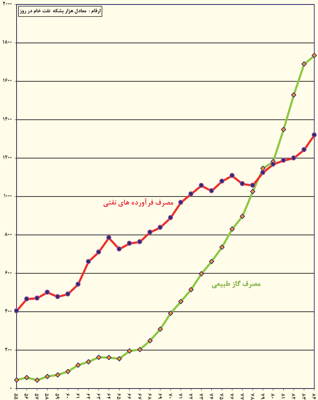
نمودار مقایسه روند مصرف گاز طبیعی با مصرف فرآورده‌های نفتی طی سال‌های ۱۳۵۵-۱۳۸۴
