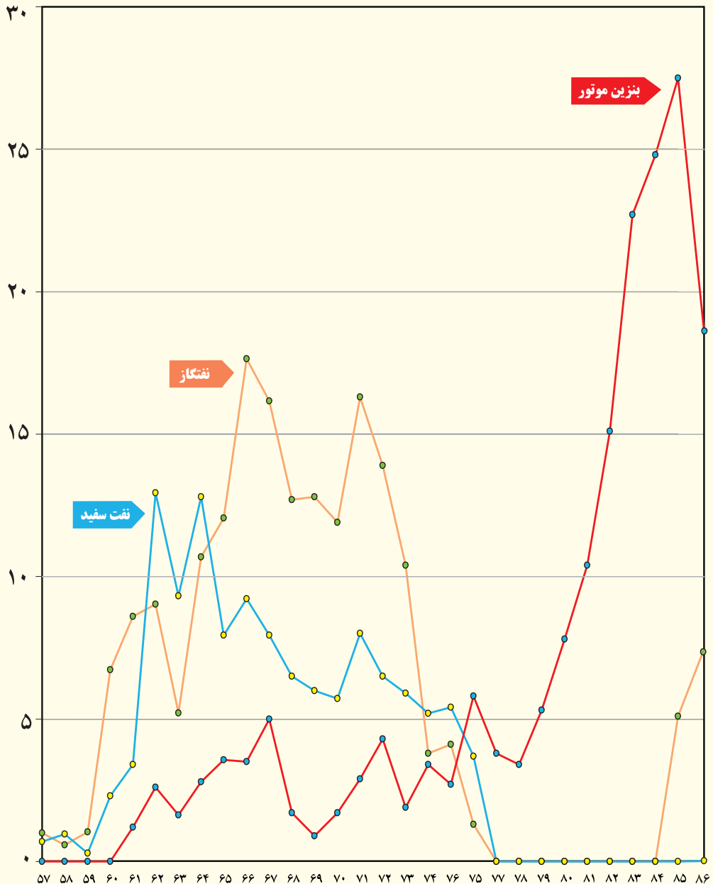
نمودار واردات بنزین موتور، نفت سفید و نفتگاز طی سالهای ۱۳۵۷-۱۳۸۶
