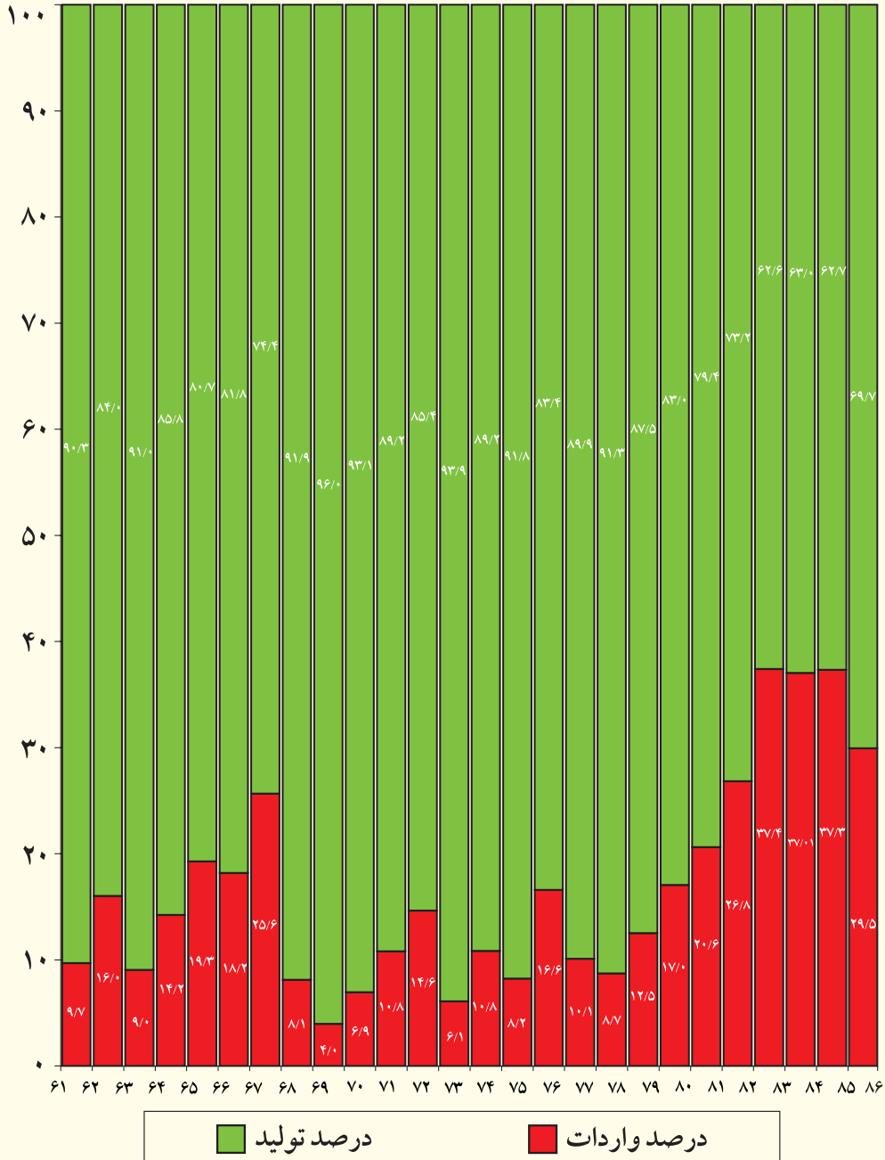
نمودار مقایسه درصد سهم واردات و تولید بنزین موتور از کل نیاز کشور طی سالهای ۱۳۶۱-۱۳۸۶
